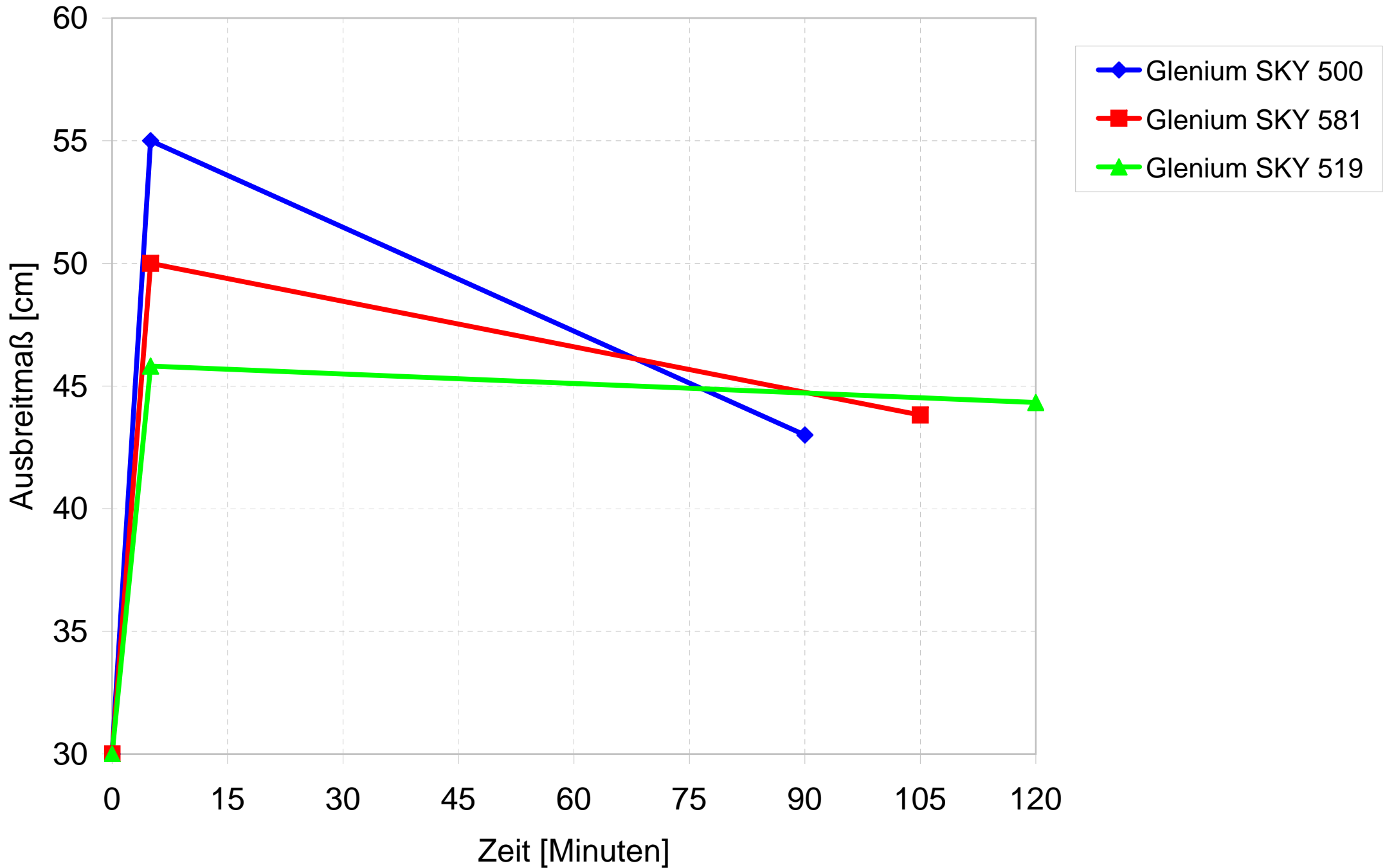
Idealisierte Darstellung der Konsistenzentwicklung von Frischbeton mit unterschiedlichen Glenium SKY Typen
